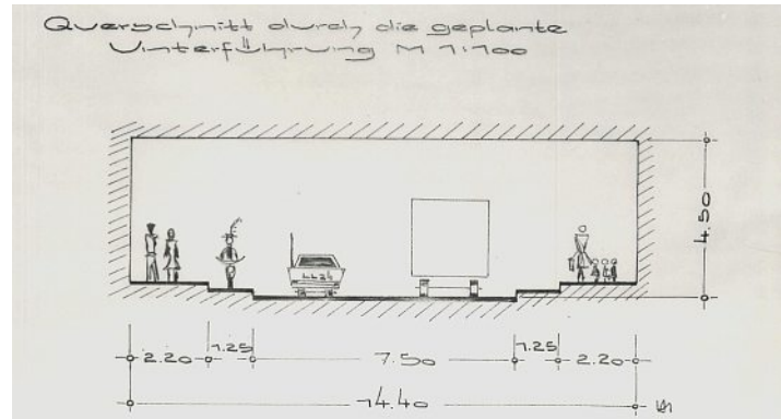
Querschnittsskizze zur neuen Unterführung, 1968.
